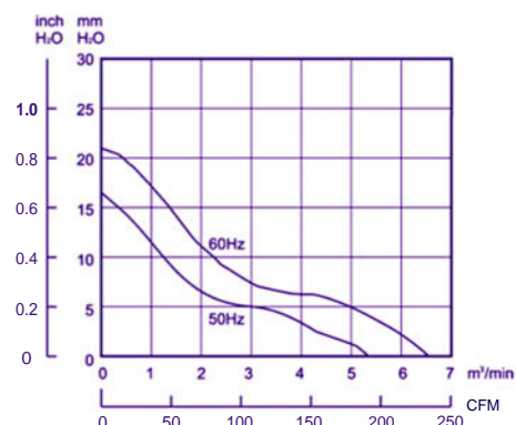
Curva de rendimiento del ventilador
